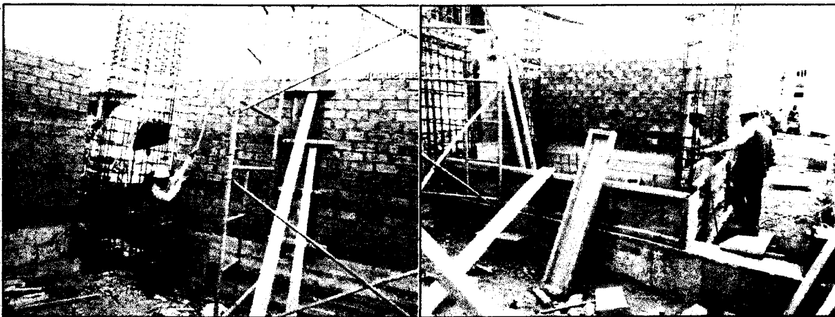
Foto N° 23 y 24: vista de los trabajos de construcción de muros de ladrillo y continuación de de encofrado de sobrecimiento así como colocación de columnetas.
