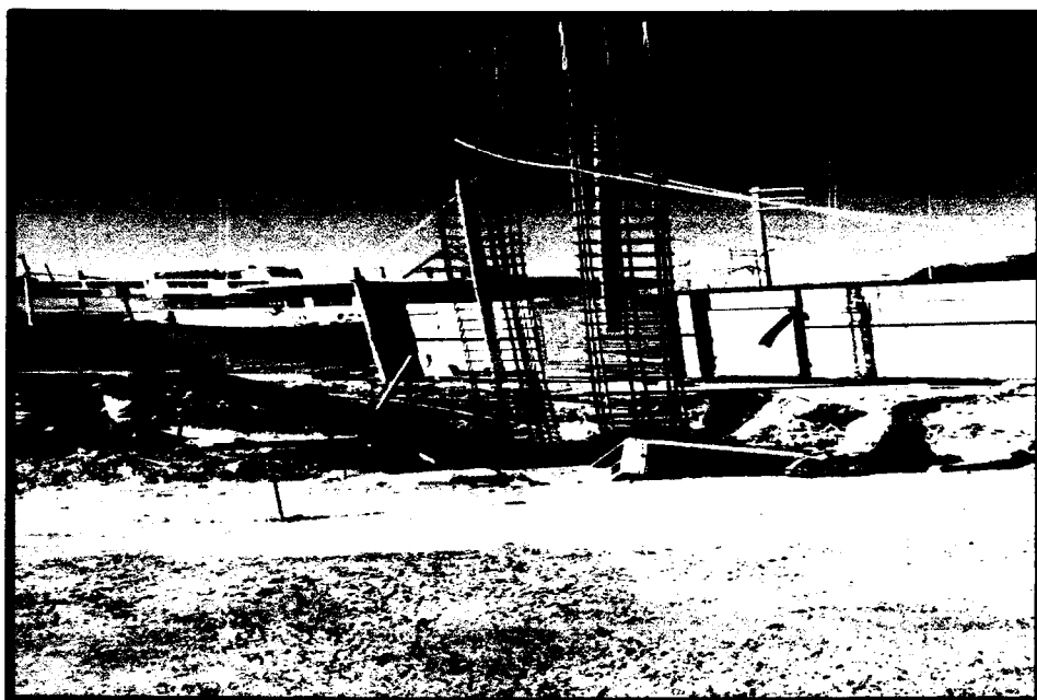
FOTOGRAFIA 01: Trabajo en área de administración.
